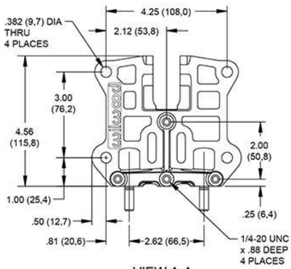
VIEW A-A
